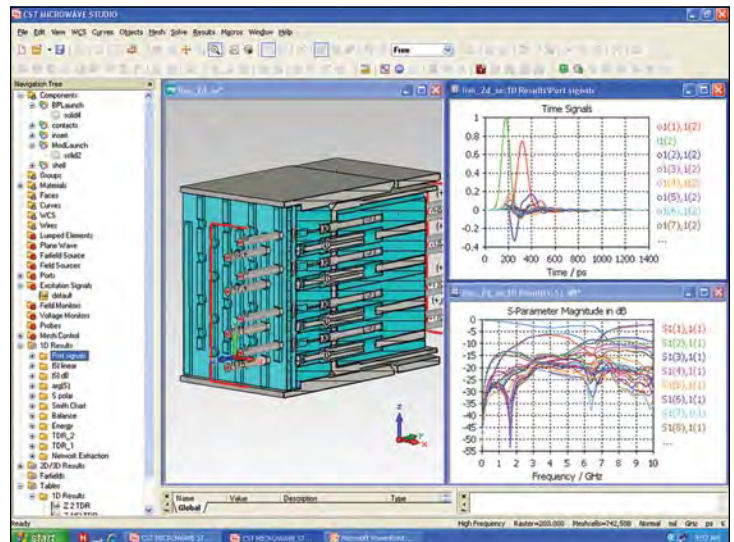
3DEM Model/S-Parameter
