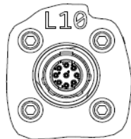
DETAIL E L1 THRU L11 10-646401-751N SCALE 1.500
