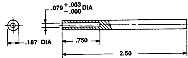
PUSH ROD
